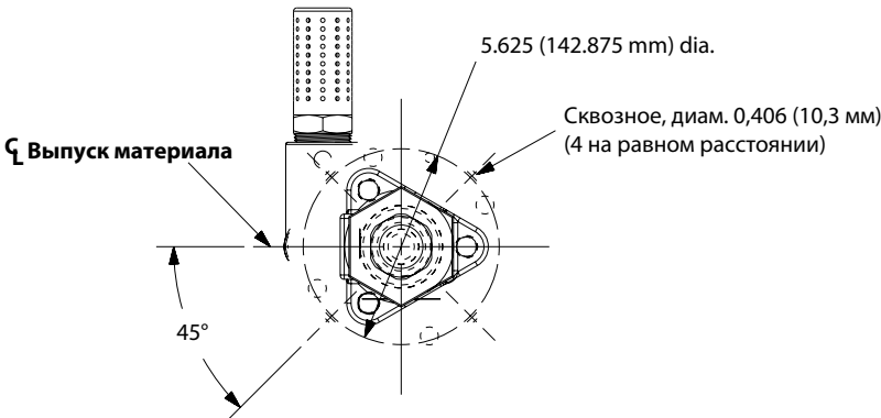
ВИД СНИЗУ
